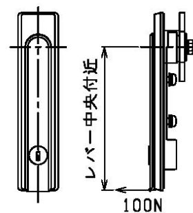
(d)平面型ハンドルスイングタイプ
