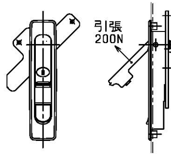
(c)平面型ハンドルリフトタイプ
