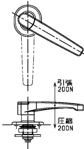
(a)レバーハンドル L 型タイプ
