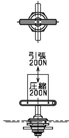
(e)抜差しハンドル正面抜差しタイプ
