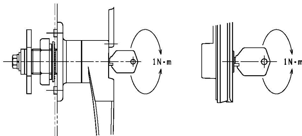
(a)レバーハンドル L 型タイプ
