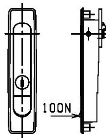
(c)平面型ハンドルフットタイプ
