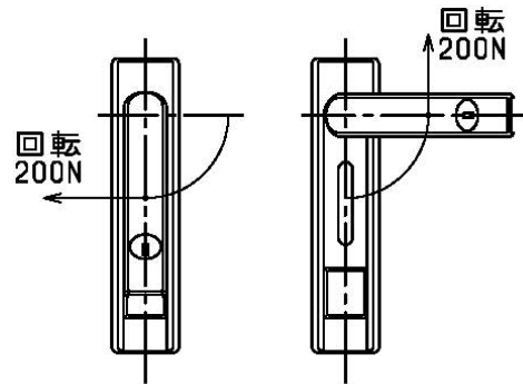
(d)平面型ハンドルスイングタイプ
