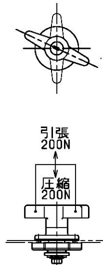
(b)レバーハンドル T 型タイプ
