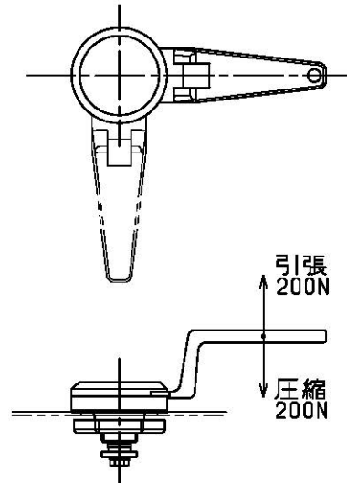
(f)抜差しハンドル下抜差しタイプ
