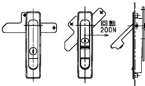
(c)平面型ハンドルリフトタイプ
