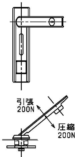
(d)平面型ハンドルスイングタイプ
