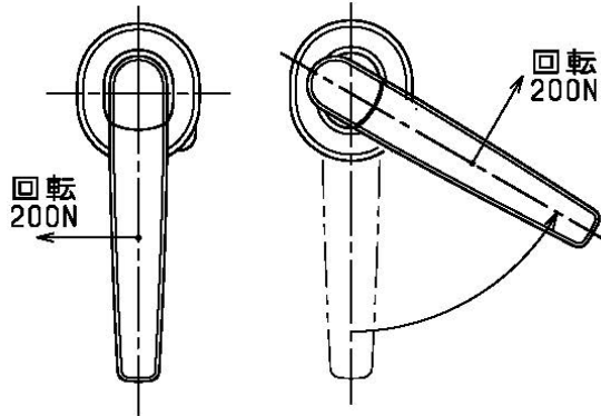
(a)レバーハンドルL型タイプ
