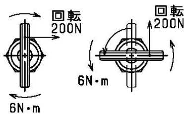
(e)拔差しハンドル正面拔差しタイプ
