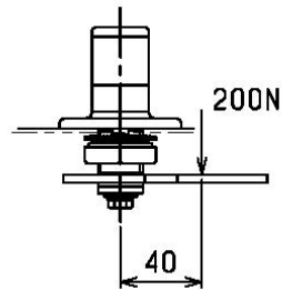
(a)レバーハンドル L 型タイプ
