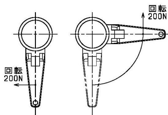
(f)拔差しハンドル下拔差しタイプ
